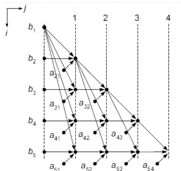
Рис. 32. Граф для алгоритму зворотної підстановки (9) для трикутної системи
