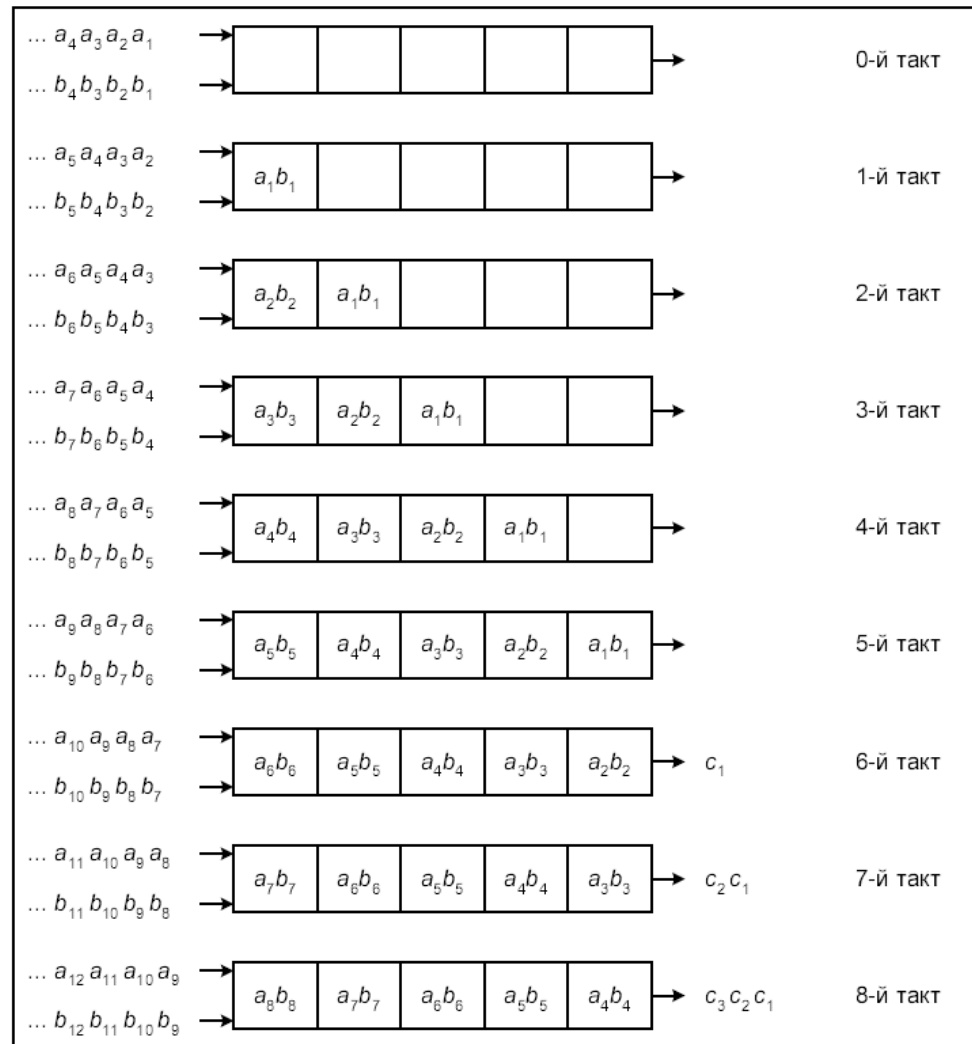
Рис. 22. Знаходження суми c = a + b за допомогою 5-стадійного конвеєрного пристрою
