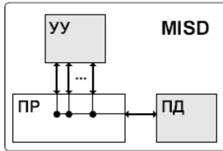
Рис. 28. Клас MISD класифікації Флінна
