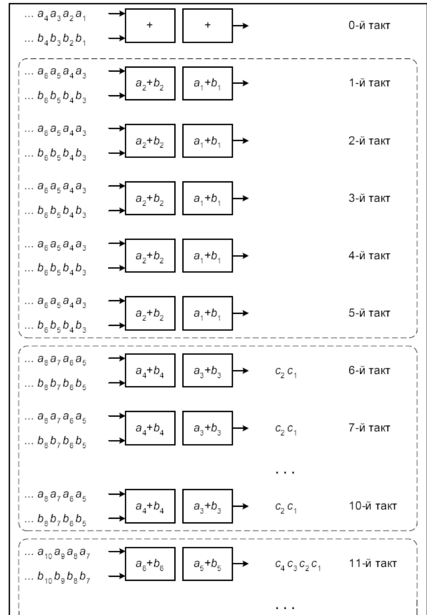
Рис. 21. Паралельне додавання векторів на двох однакових пристроях
