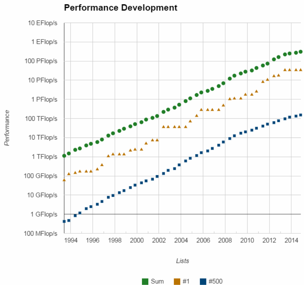
Рис. 15. Зростання продуктивності суперкомп'ютерів (за даними Top500.org ).
