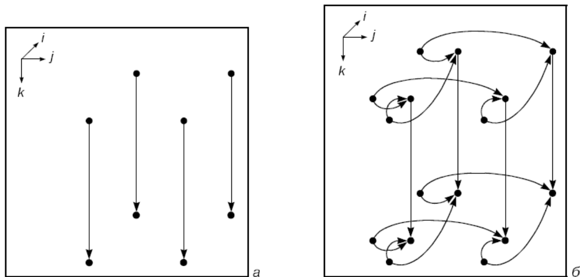
Рис. 31. Граф алгоритму множення матриць
