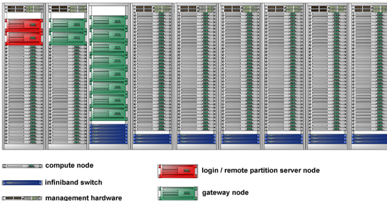
Рис. 7. Схема будови кластера LLNL
