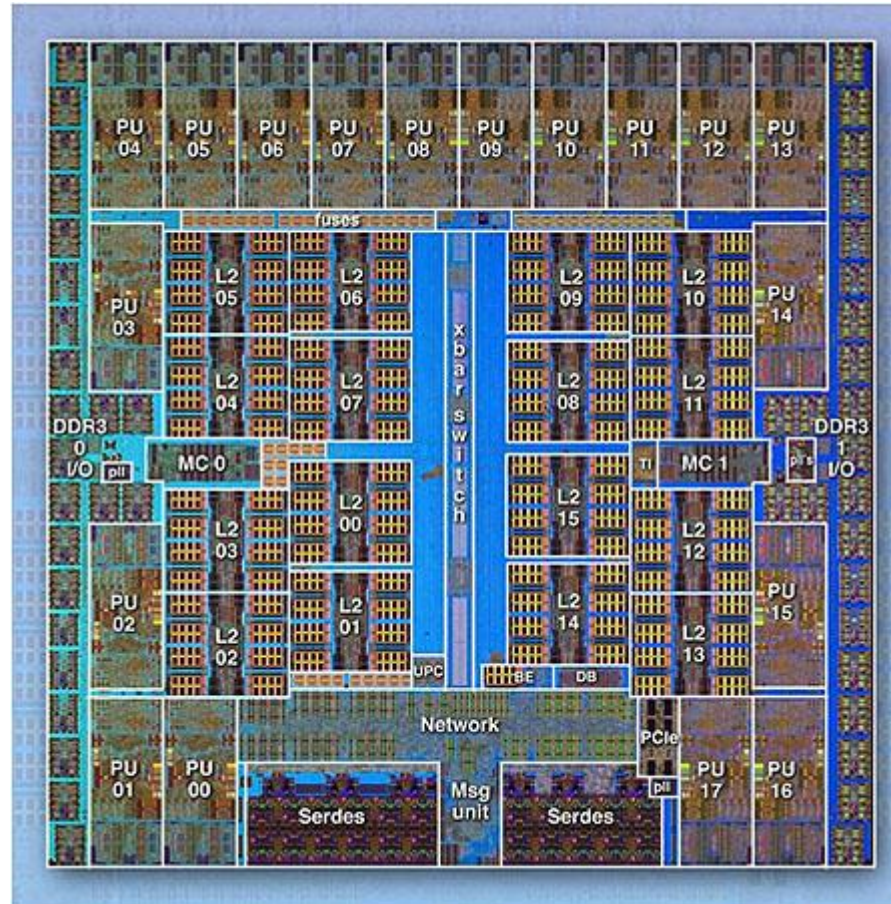
Рис. 5. Обчислювальний чіп IBM VG/Q
