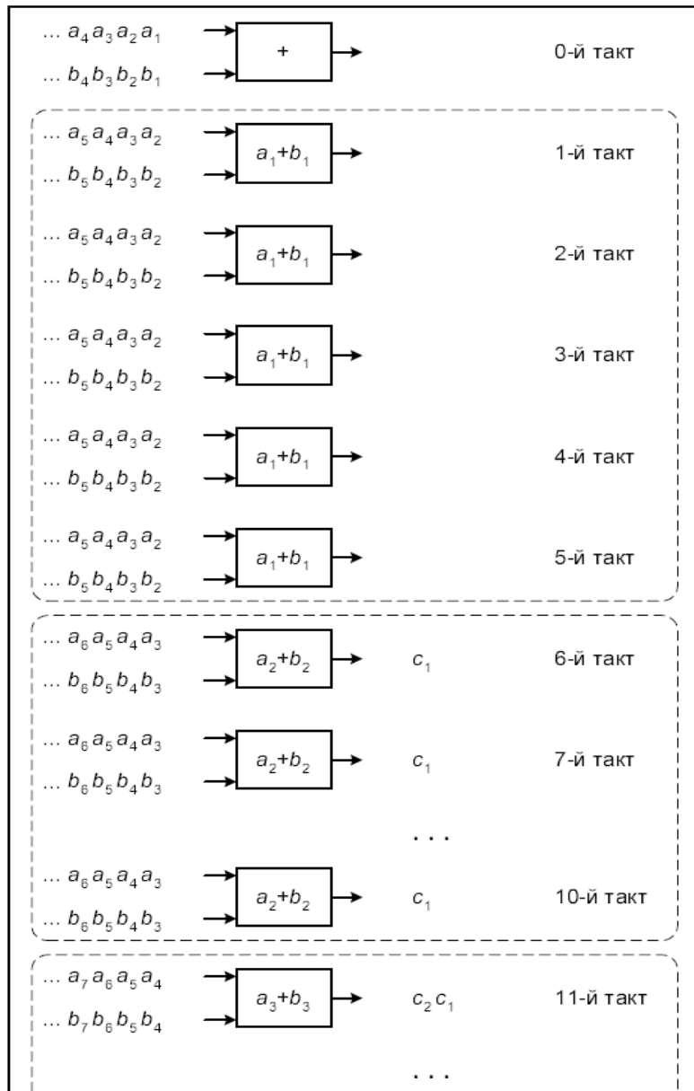
Рис. 20. Додавання векторів на послідовному пристрої з 5-тактовою операцією додавання
