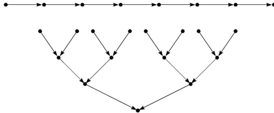
Рис. 30. Послідовний граф та граф алгоритму "здвоєння"
